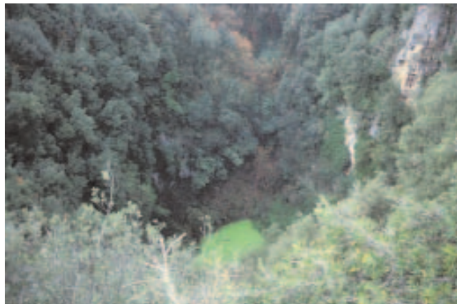
La voragine del Pozzo del Merro
